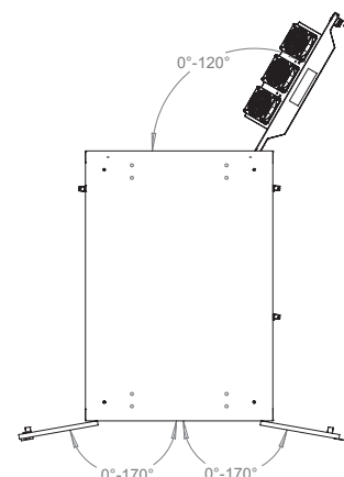
Angle d'ouverture de la porte avant
