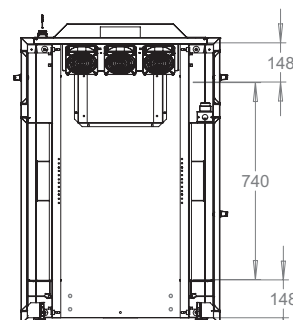
Distance d'installation de l'équipement
