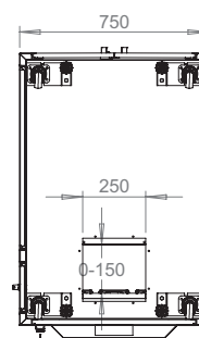
Vue du bas
