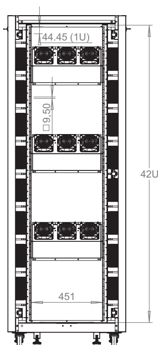
Dimensions en largeur et en hauteur
